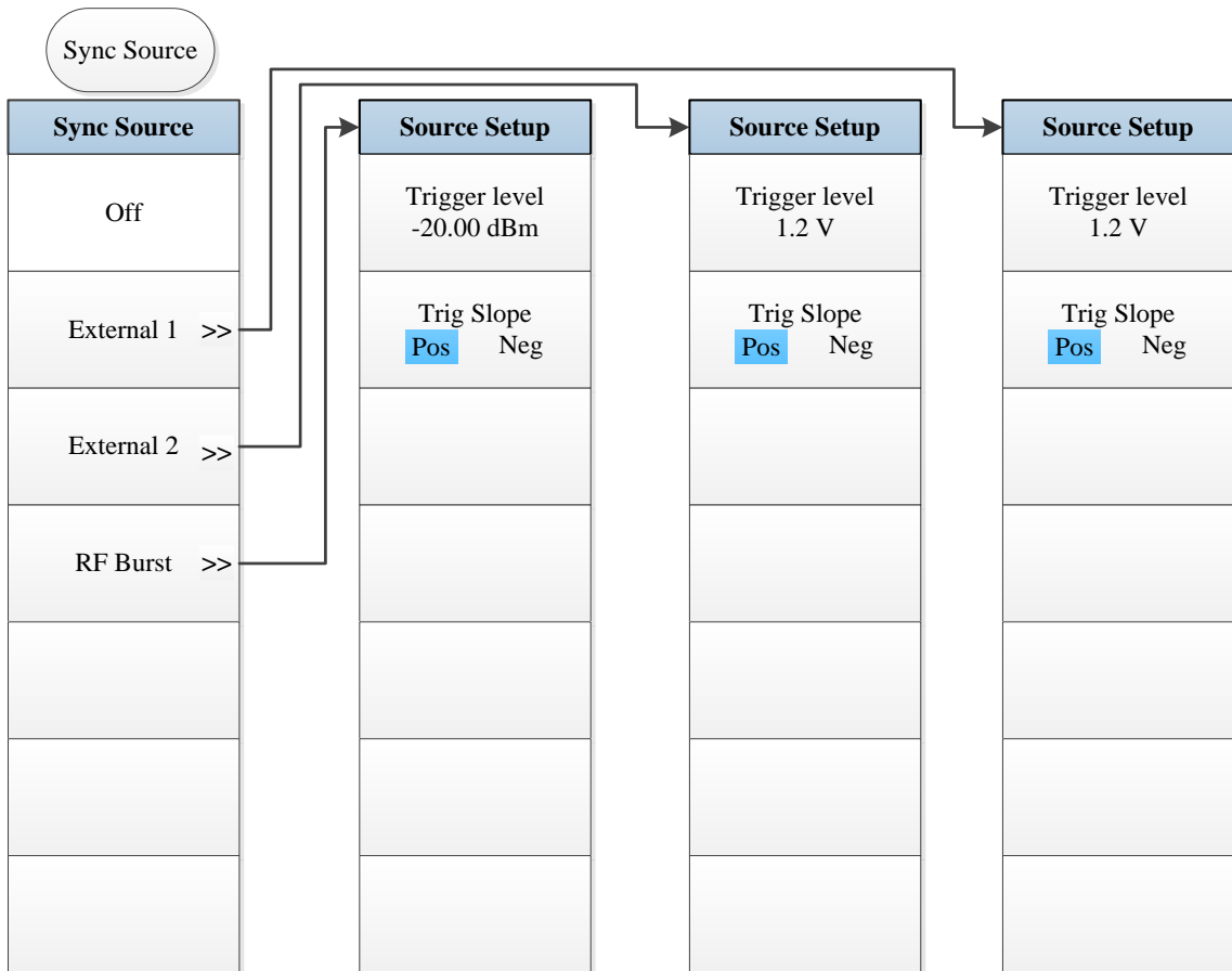
Fig. 5.5-6 Trigger Menu
