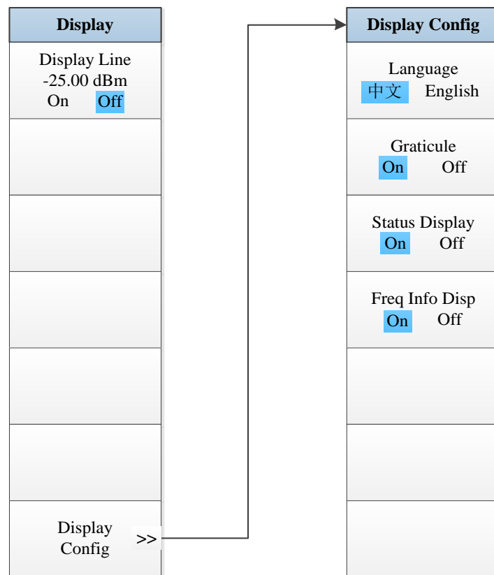
Fig. 5.6-11 Display Menu
